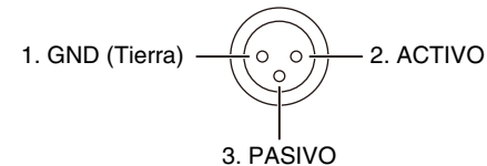
Tomas de salida XLR
